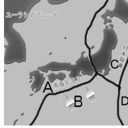
プレート構造図 (図2)
