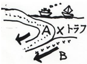
トラフで地震が起きる (図3)
